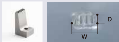
有効溶着範囲 6(W)×3(D)mm
